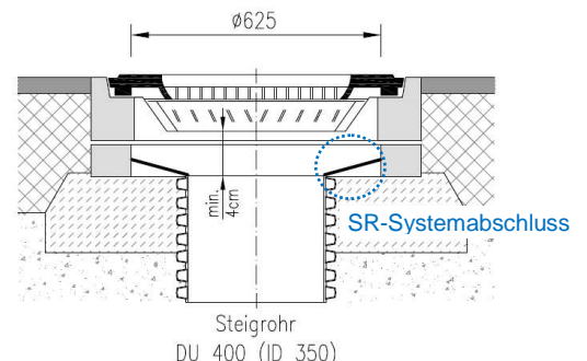
Schematischer Schnitt Abdeckung DIN 124 mit Ø 625: Lastabtrag über einen Betonring 325mm mit Betonauflager. Das Steigrohr auf Passfähigkeit zu dem Schmutzfänger kürzen und mit SR-Systemabschluss 625/350 abschließen!
