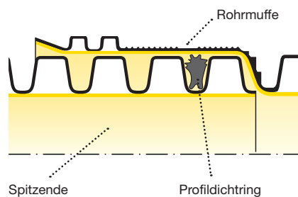
Beispiel: Rohrverbindung mit angeformter Muffe
