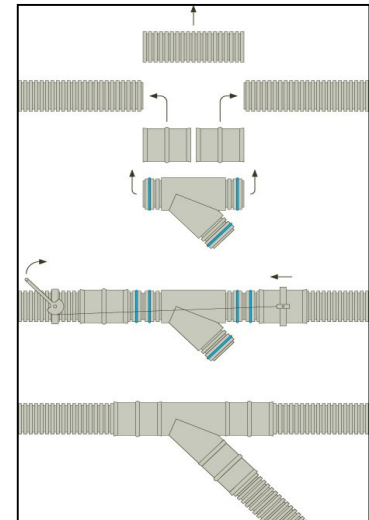
Bild 4) nachträglicher Anschluss
