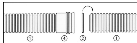
Bild 2) Rohrverbindung mit angeformter Muffe
